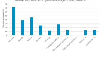
Aandeel warmteverlies, Vrijstaande woningen >1995, Niveau 4
