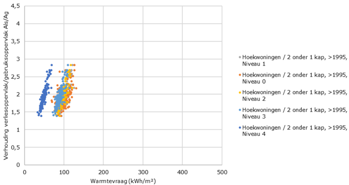
Figuur 78: netto warmtevrraag: Hoekwoningen en 2 onder 1 kapwoningen, bouwperiode na 1995
