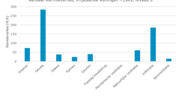
Aandeel warmteverlies, Vrijstaande woningen <1945, Niveau 3
