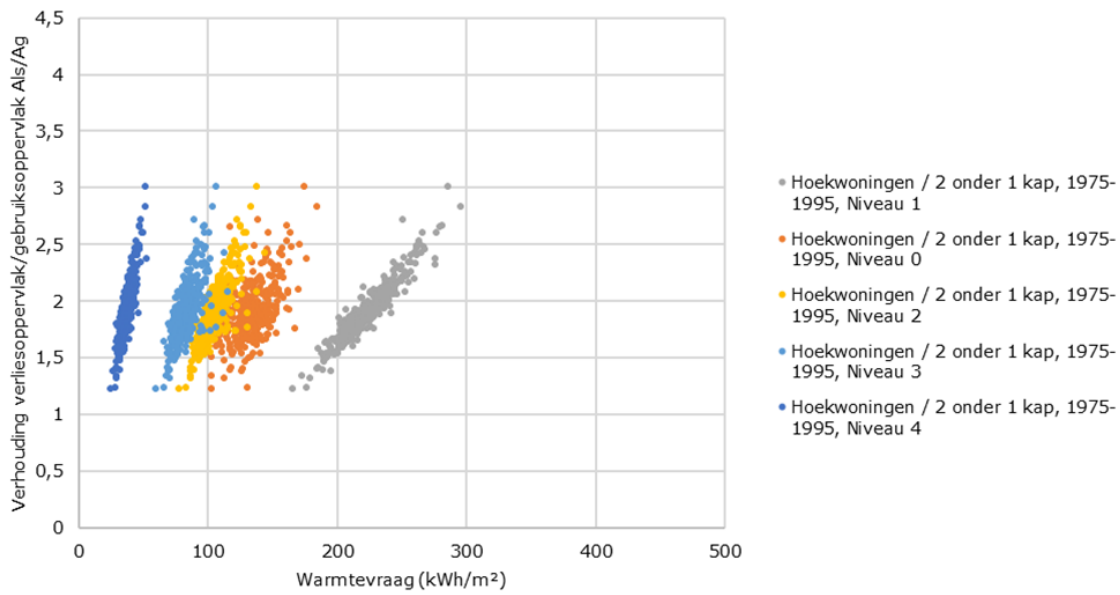
Figuur 77: netto warmtevrraag: Hoekwoningen en 2 onder 1 kapwoningen, bouwperiode 1975-1995
