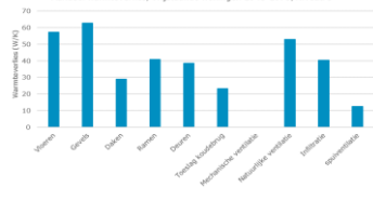
Aandeel warmteverlies, Vrijstaande woningen 1945-1975, Niveau 3
