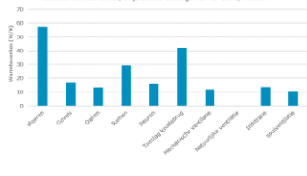
Aandeel warmteverlies, Vrijstaande woningen 1945-1975, Niveau 4
