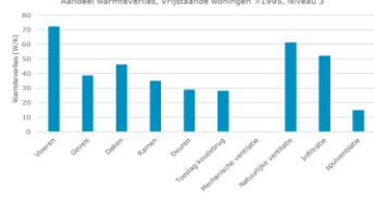
Aandeel warmteverlies, Vrijstaande woningen >1995, Niveau 3
