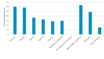
Aandeel warmteverlies, Vrijstaande woningen 1975-1995, Niveau 3
