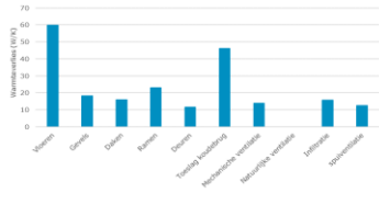
Aandeel warmteverlies, Vrijstaande woningen 1975-1995, Niveau 4
